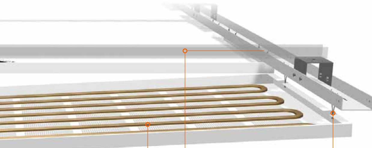
Apertura SafeSystem e bugne di autocentraggio SafeSystem opening and self-centering clues E
