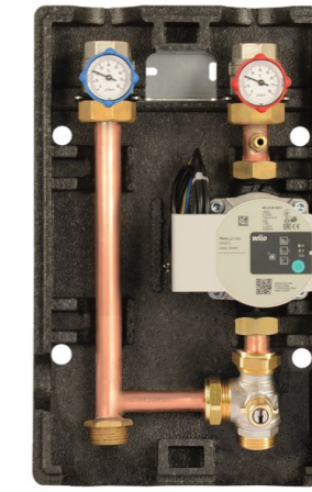
Gruppo di regolazione climatica
