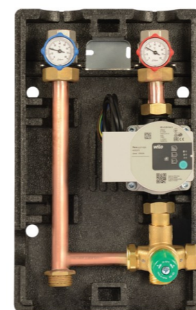
Gruppo di regolazione punto fisso
