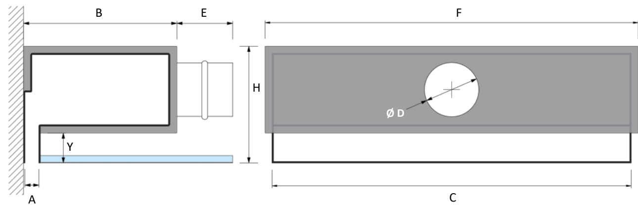
Dimensioni dei diffusori lineari TRATTO P | Dimensions of TRATTO P linear diffusers
