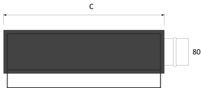
attacco di testa | head connector
